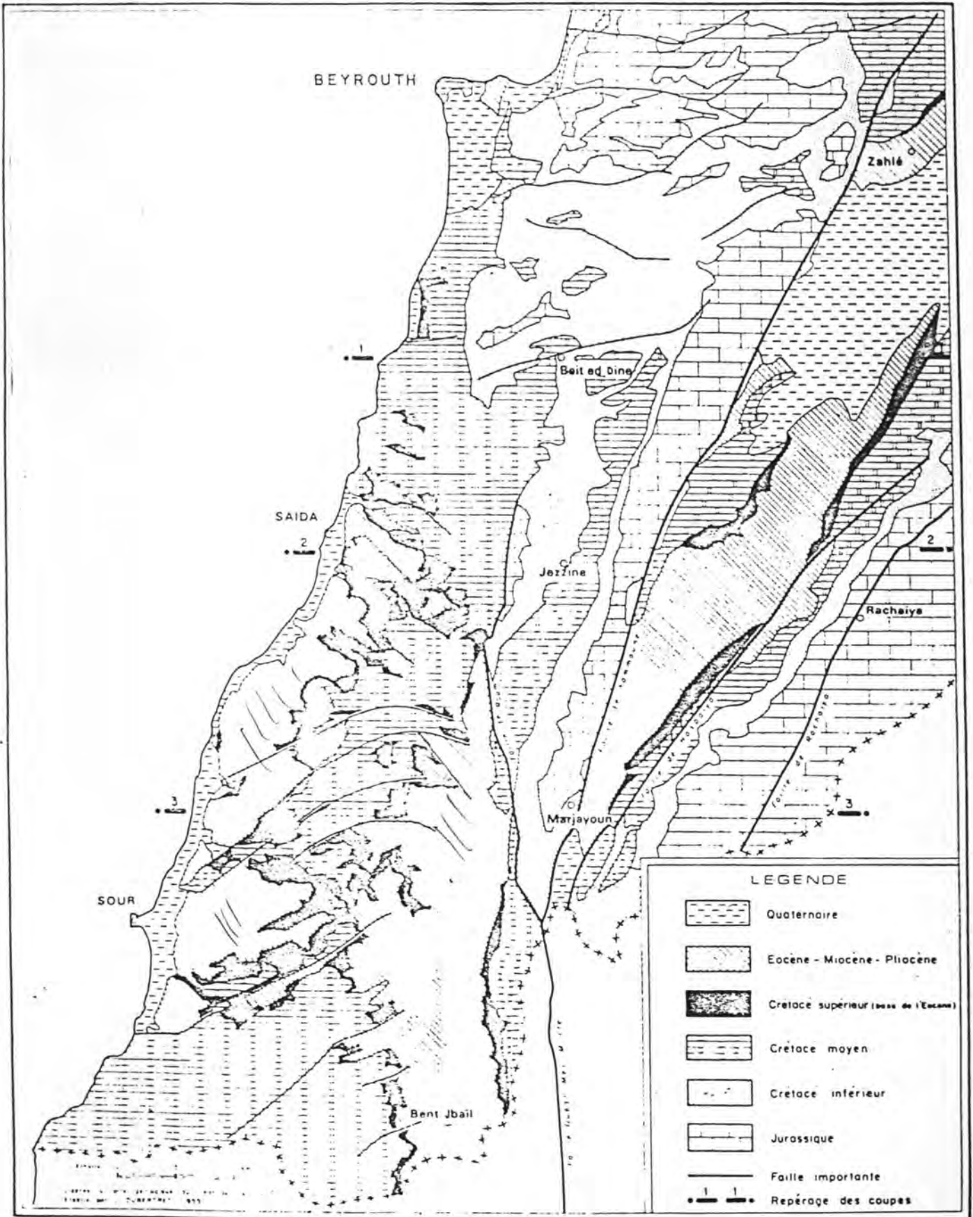
GÉOLOGIE RÉGIONALE
